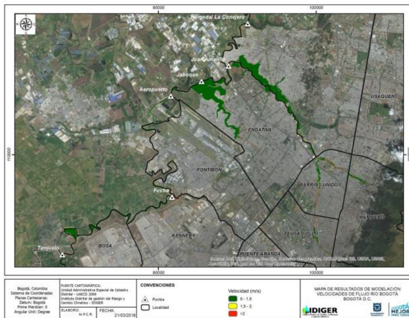
Figura 5 Resultados de la modelación del río Bogotá (Velocidades de flujo)
