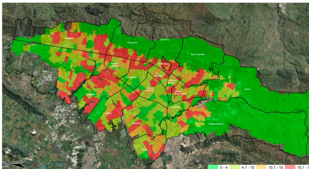
Figura 9 Densidad de eventos por encharcamiento
