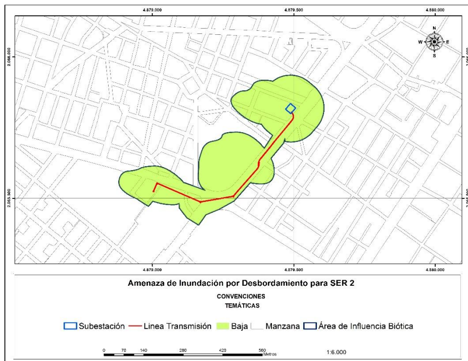
Figura 7 Amenaza de inundación para el área de estudio
