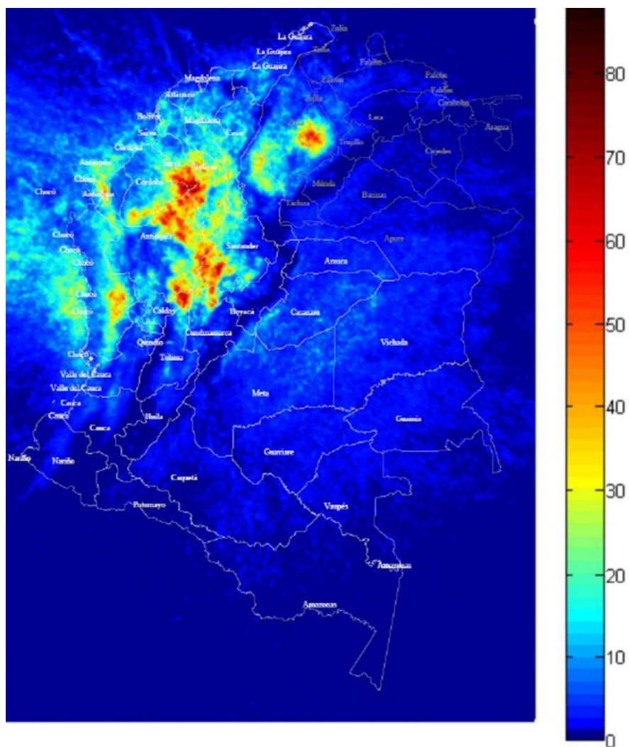
Figura 12 Mapa de densidad de rayos en Colombia para el año 2012
