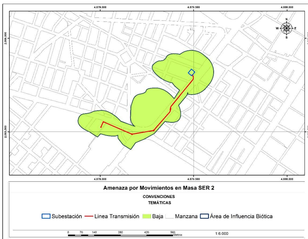
Figura 4 Amenaza sísmica del área de estudio
