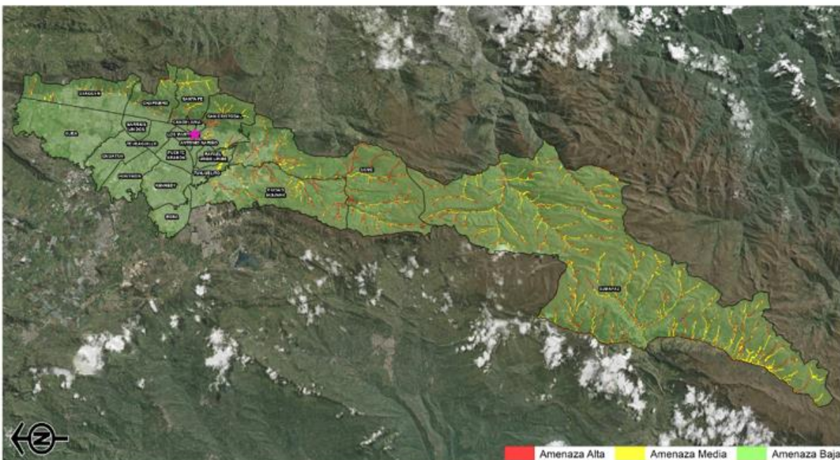
Figura 8 Zonificación de amenaza por avenidas torrenciales
