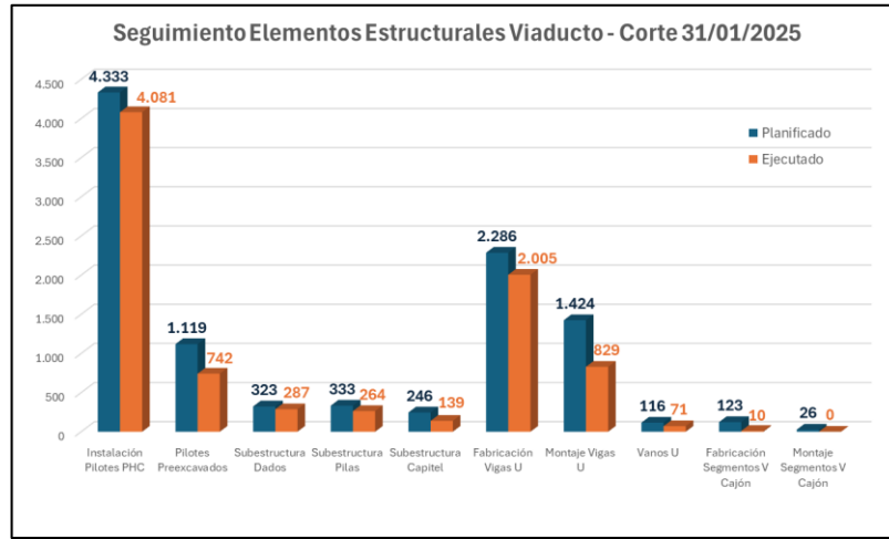
Figura 3.2-3. Seguimiento Elementos Estructurales del viaducto – Corte 31/01/2025
