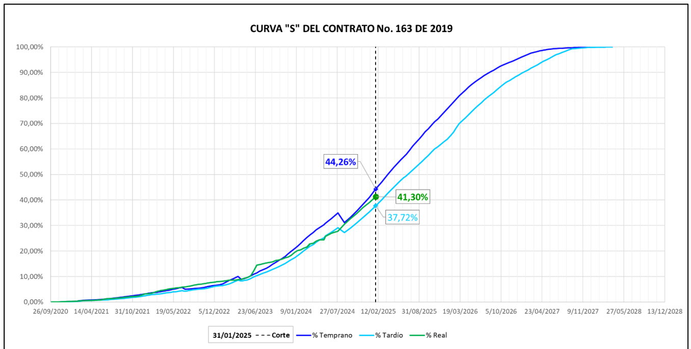
Figura 3.3-2. Avance general del Proyecto PLMB con % programado PEV12 Vs % ejecutado – Corte 31/01/2025
